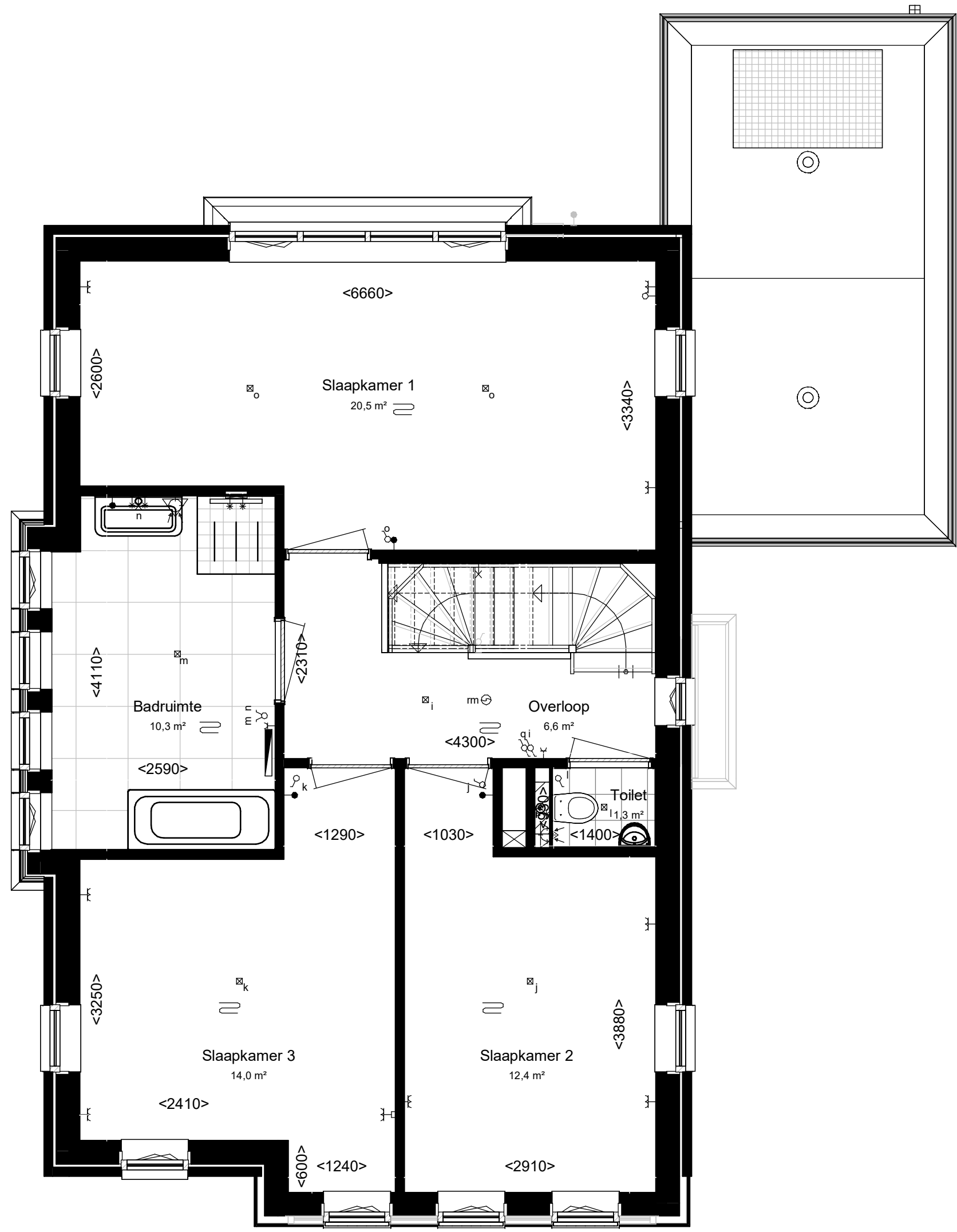
Eerste verdieping, 2960+P
