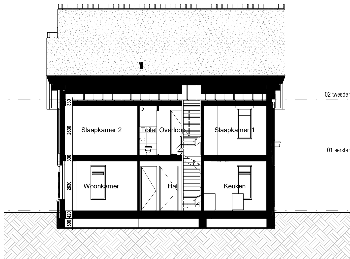
Doorsnede (1:100)
