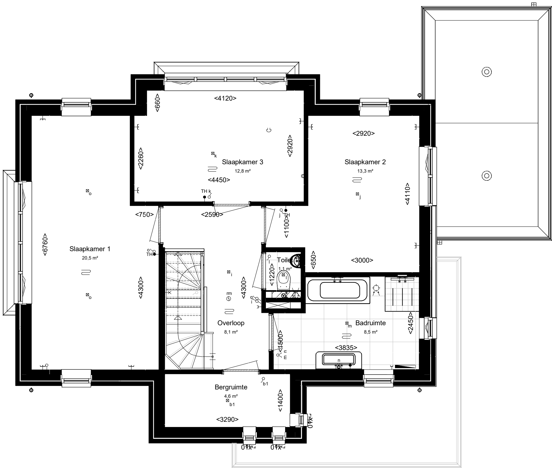
Eerste verdieping, 2960+P
