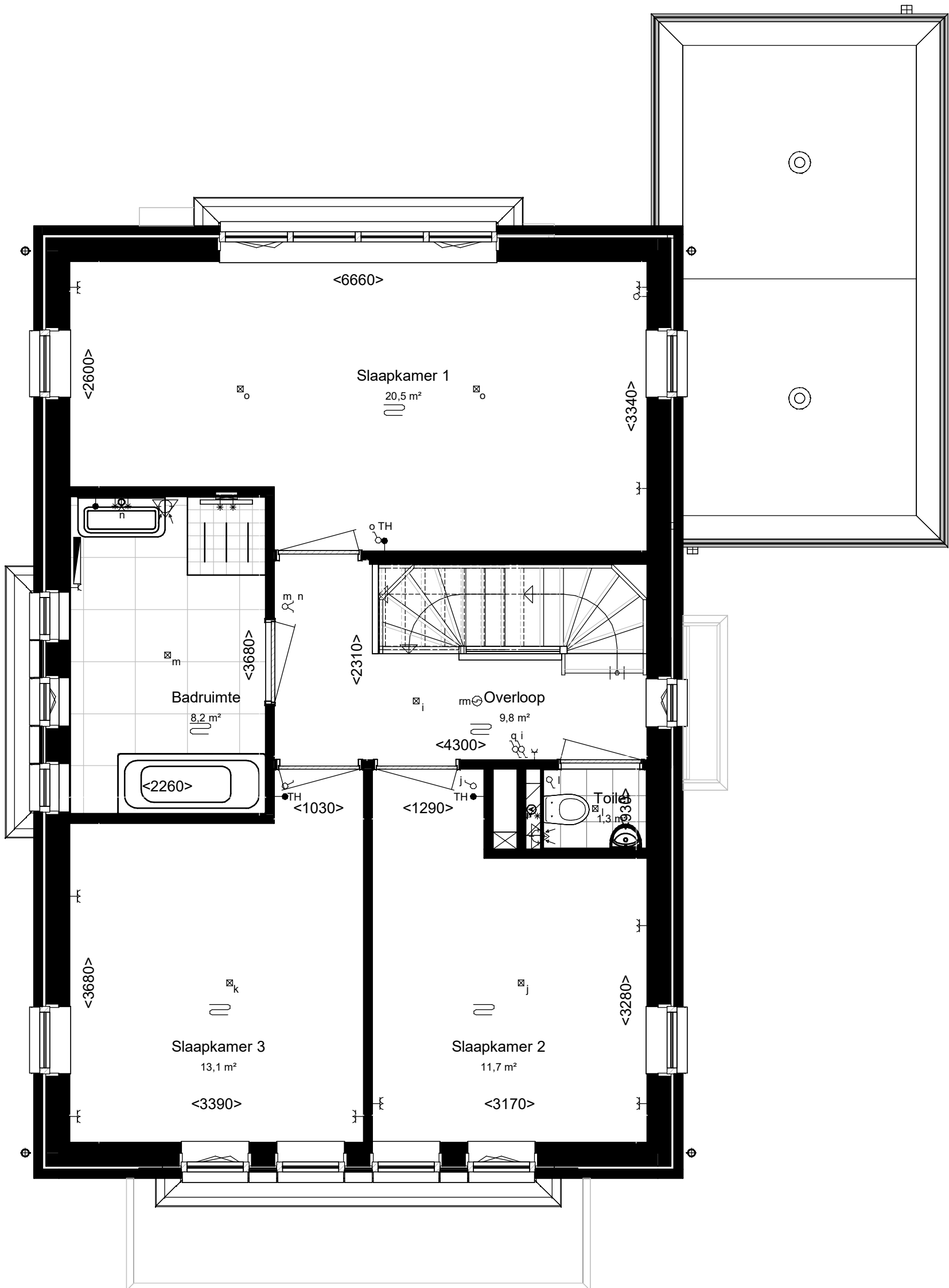
Eerste verdieping, 2960+P
