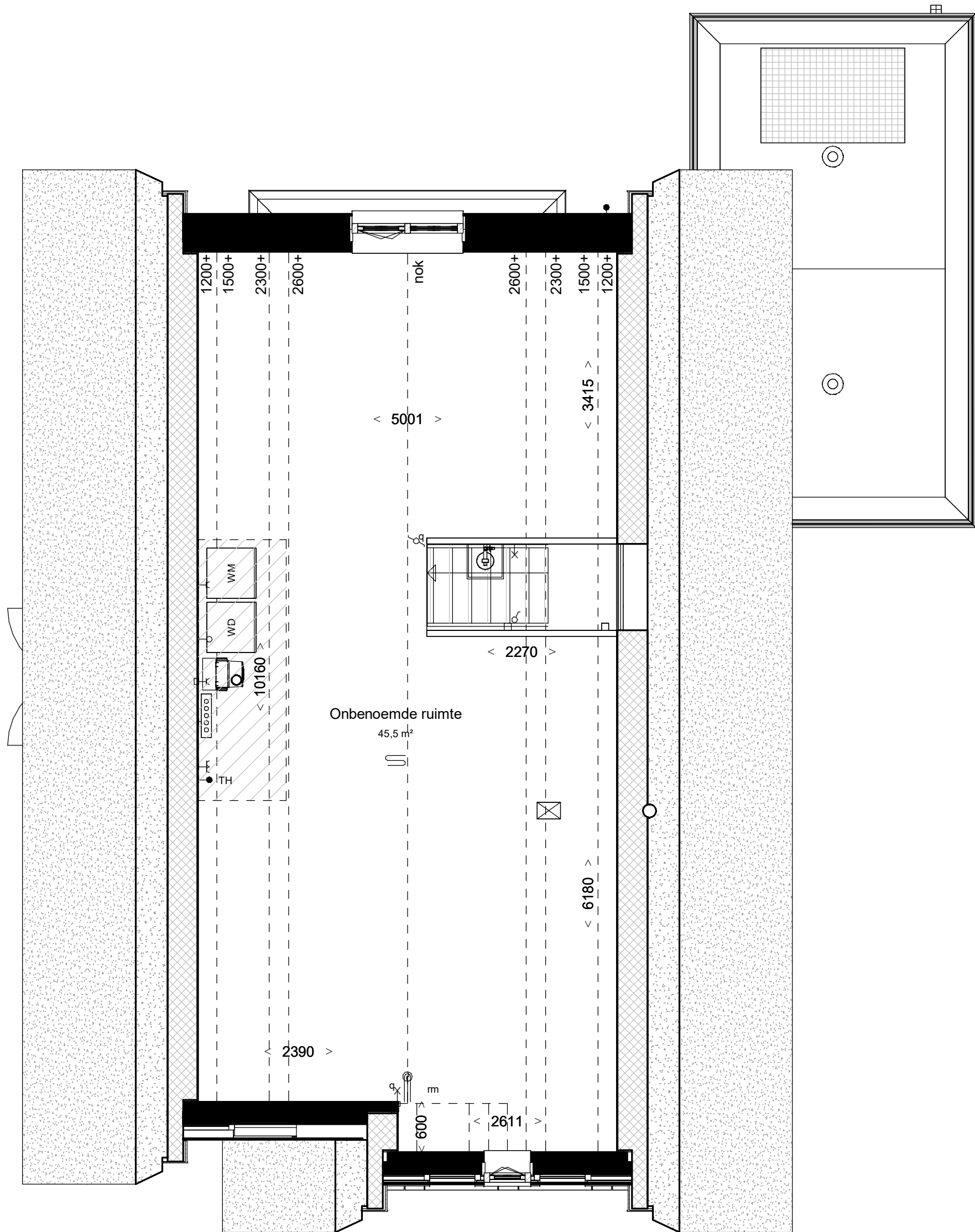
Tweede verdieping 5920+P
