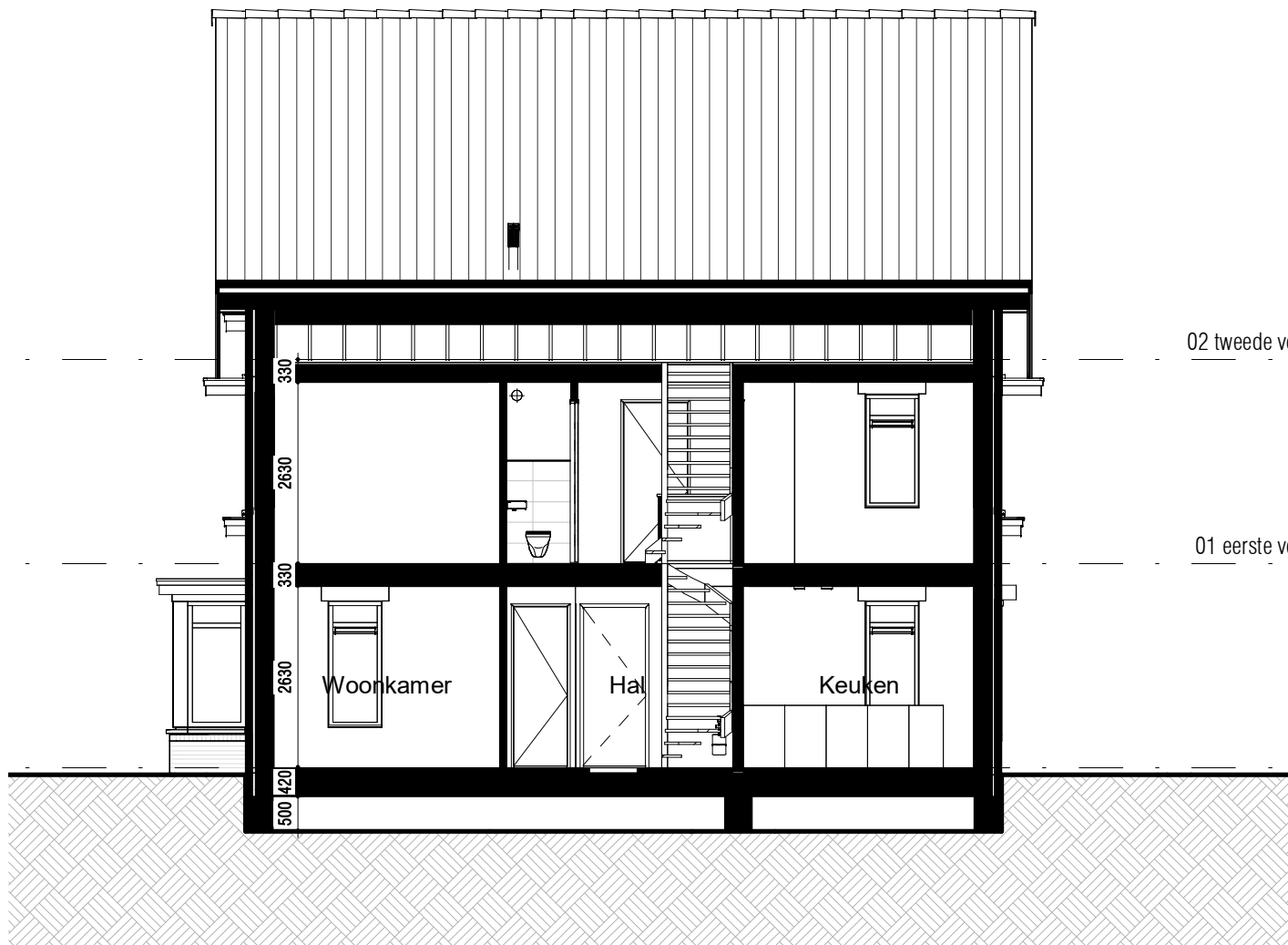
Doorsnede (1:100)
